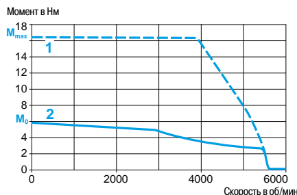
С сервопреобразователем LXM 32●D30M2
