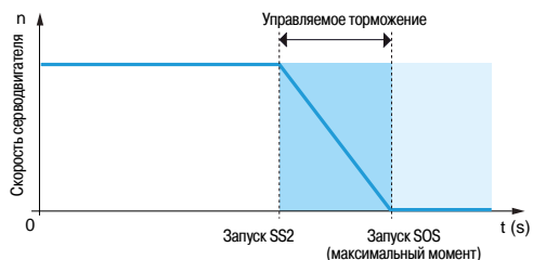
Запуск функции безопасности "Safe Stop 2" (SS2)
