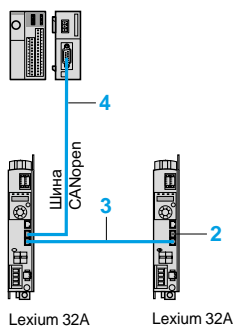
Пример архитектуры с управлением от ПЛК Twido
