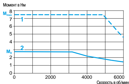
С сервопреобразователем LXM 32●D18M2
